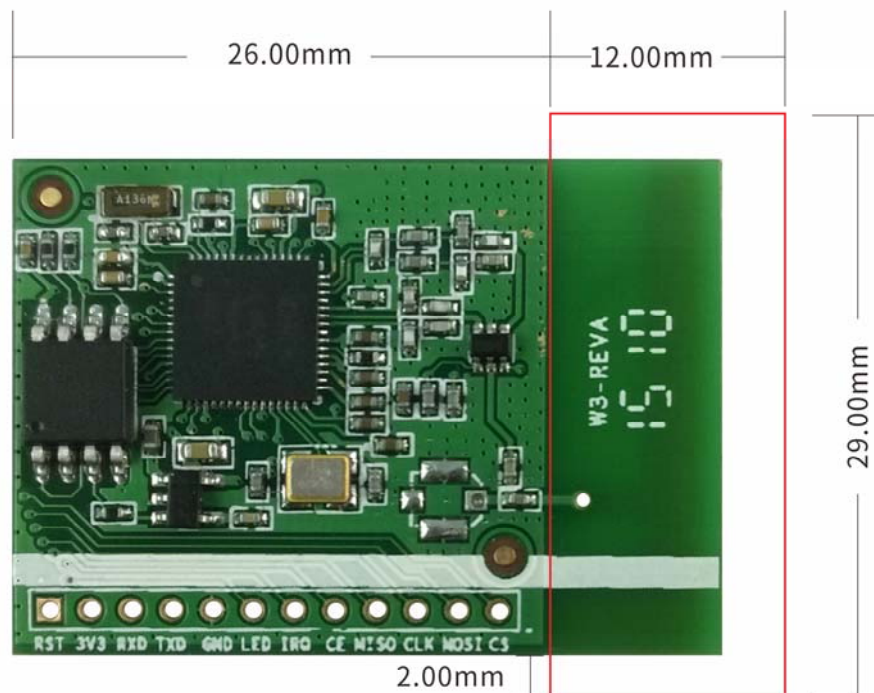
图 1-3 iWulink W301-1.0 禁布区尺寸
