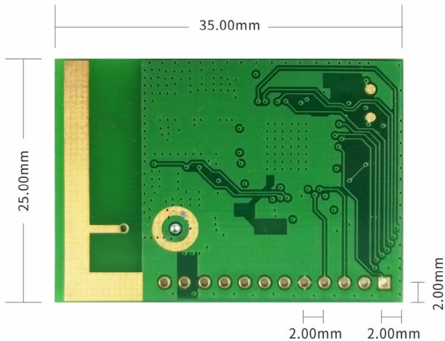
图 1-3 iWulink W301-1.0 禁布区尺寸
