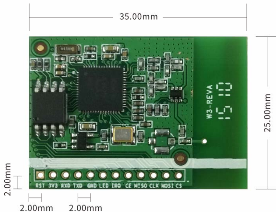
图 1-1 iWulink W301-1.0 正面
