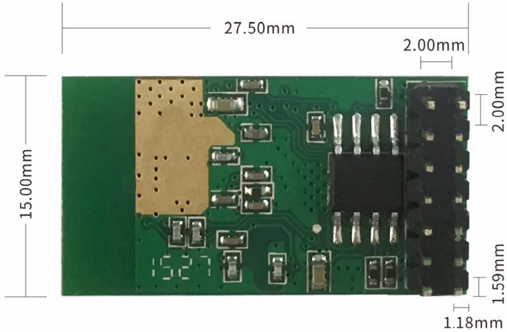
图 1-3 iWulink W402-1.0 天线区域尺寸
