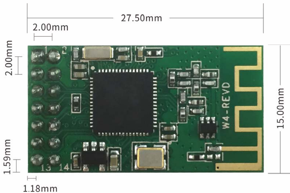
图 1-1 iWulink W402-1.0 正面
