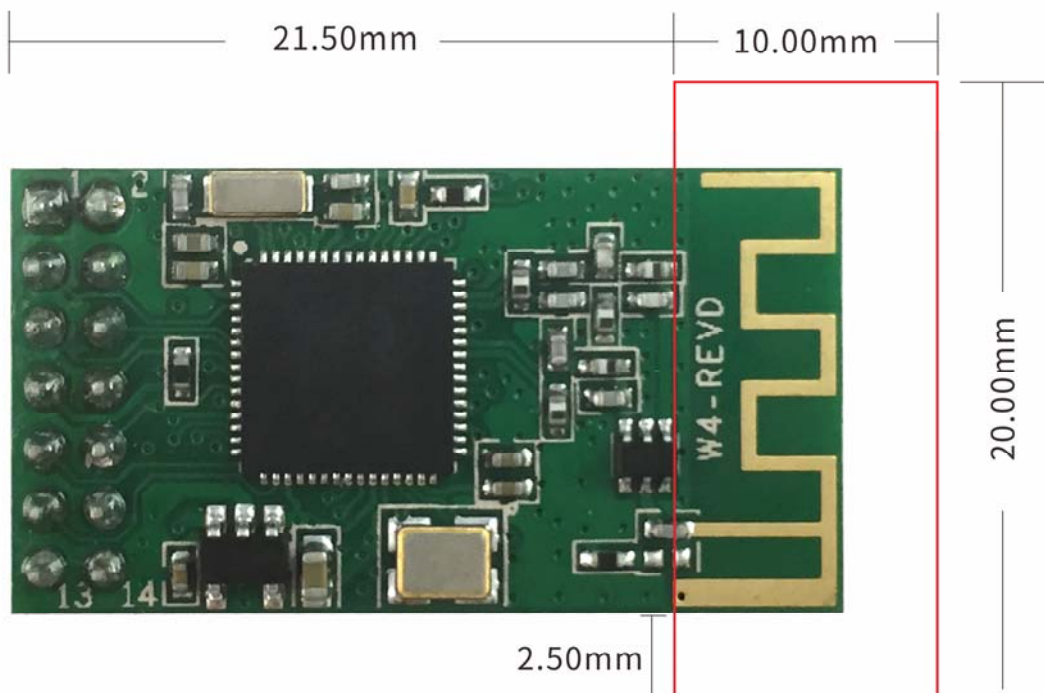
图 1-3 iWulink W402-1.0 天线区域尺寸
